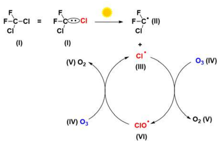
Esquema 2. Destrucción del ozono por radicales cloro provenientes de los clorofluorocarbonos.
