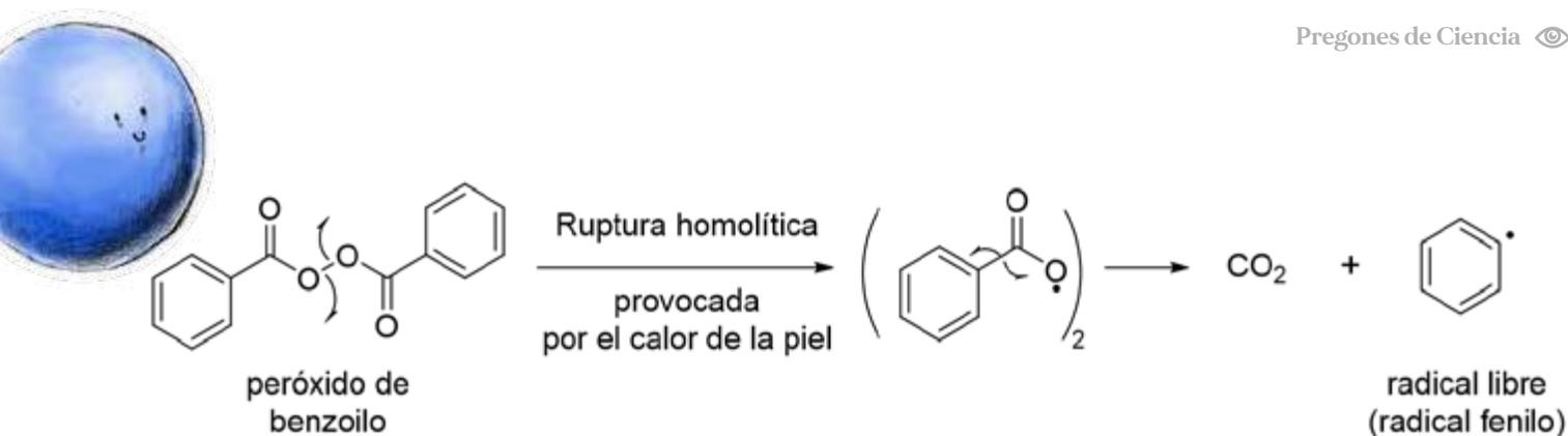
Esquema 4. Ruptura homolítica del peróxido de benzoilo.
