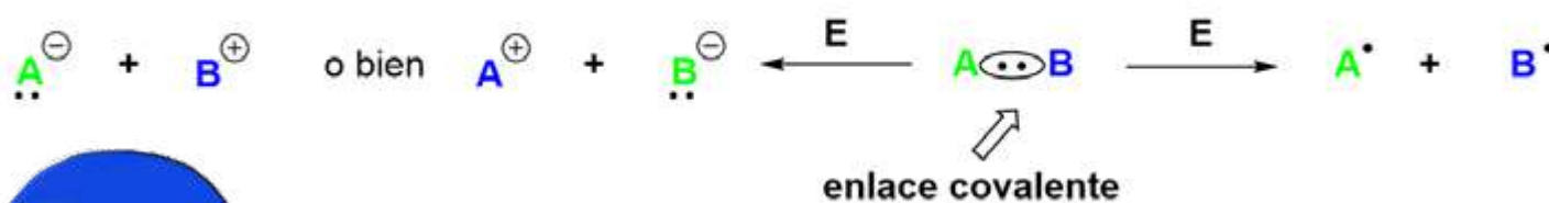
Esquema 1. Formación de iones y de radicales libres dependiendo del tipo de ruptura de una molécula A-B.
